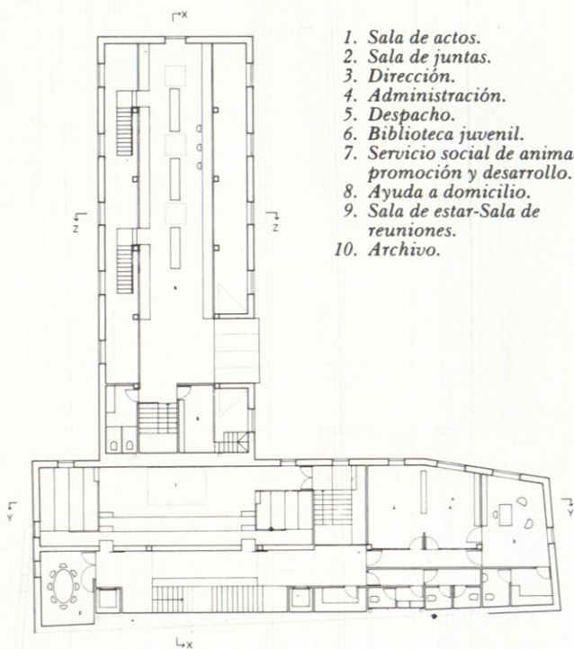
PLANTA SEGUNDA
