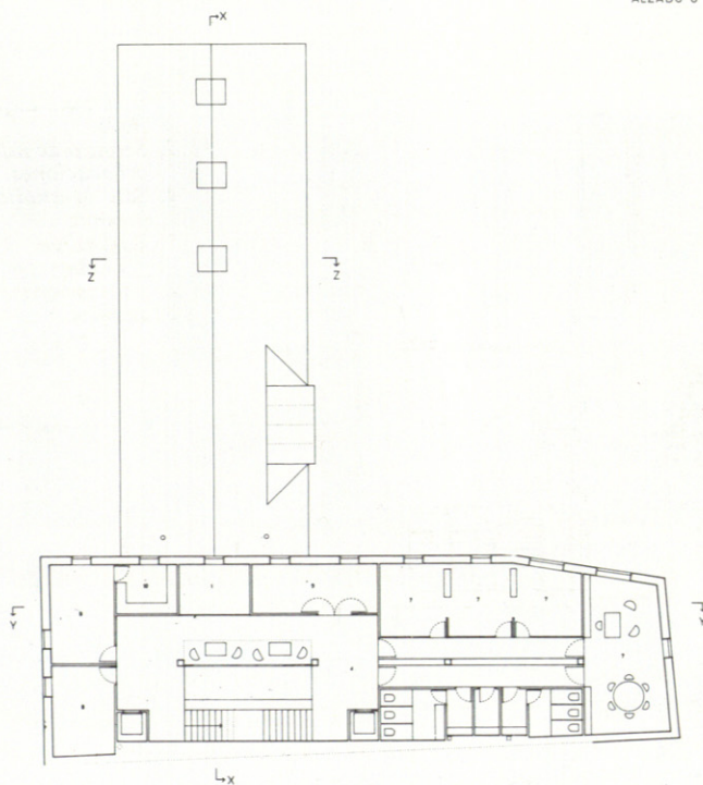
PLANTA TERCERA
